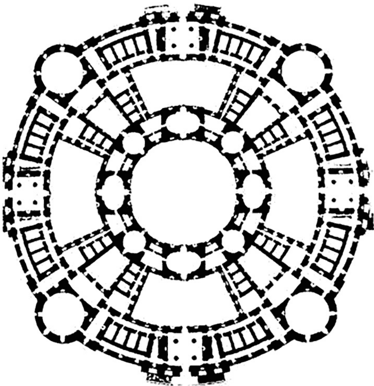
LÁMINA 15. Plano de la Galera de Gante, 1773. Cf. p. 126.
