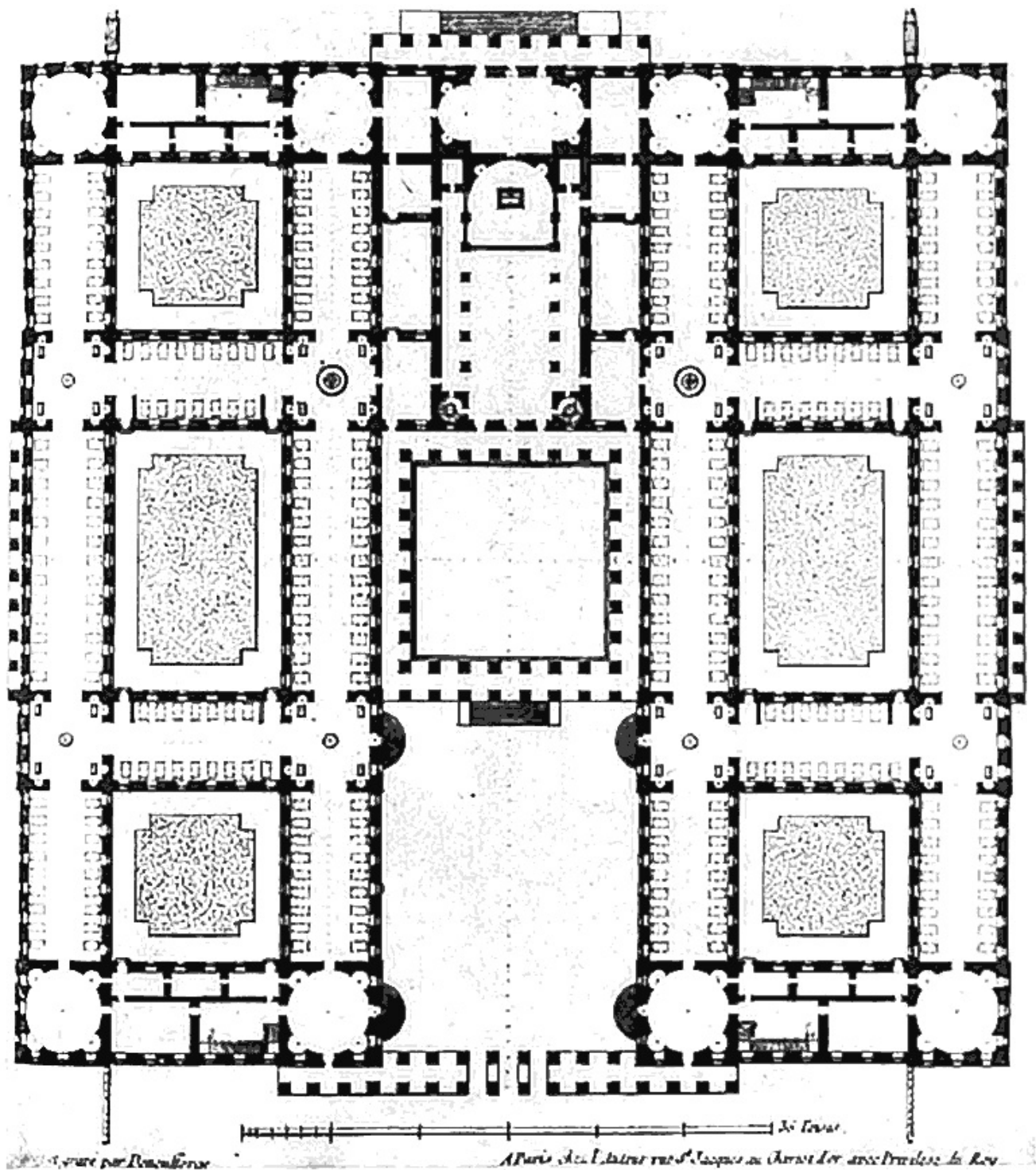
LÁMINA 13. J. F. de Neufforge. Proyecto de hospital. Colección elemental de arquitectura (1757-1780). Cf. p. 179.
